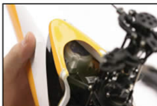
14.将陀螺仪安装好 Assemble the gyro.
